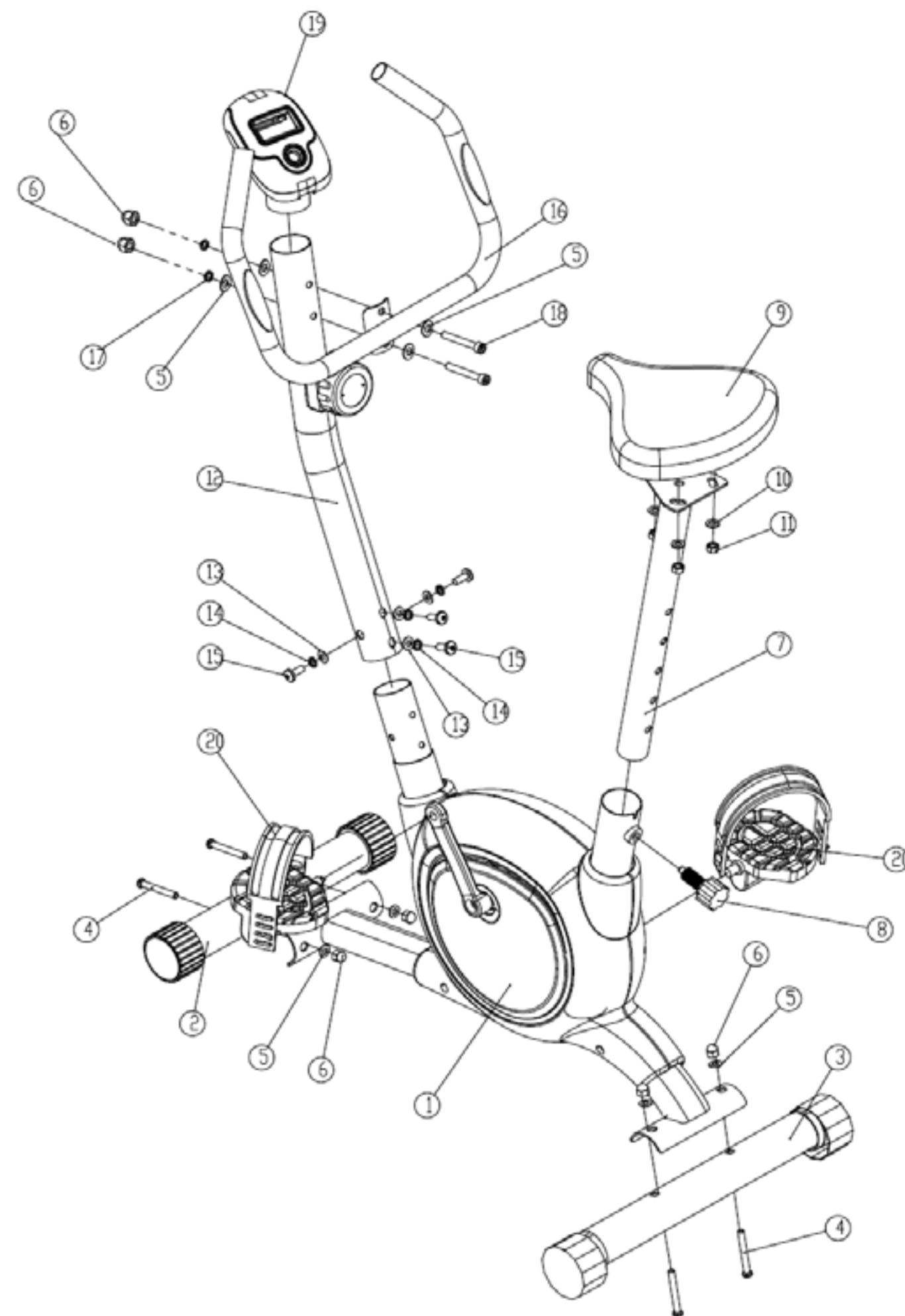
РИСУНОК-СХЕМА
