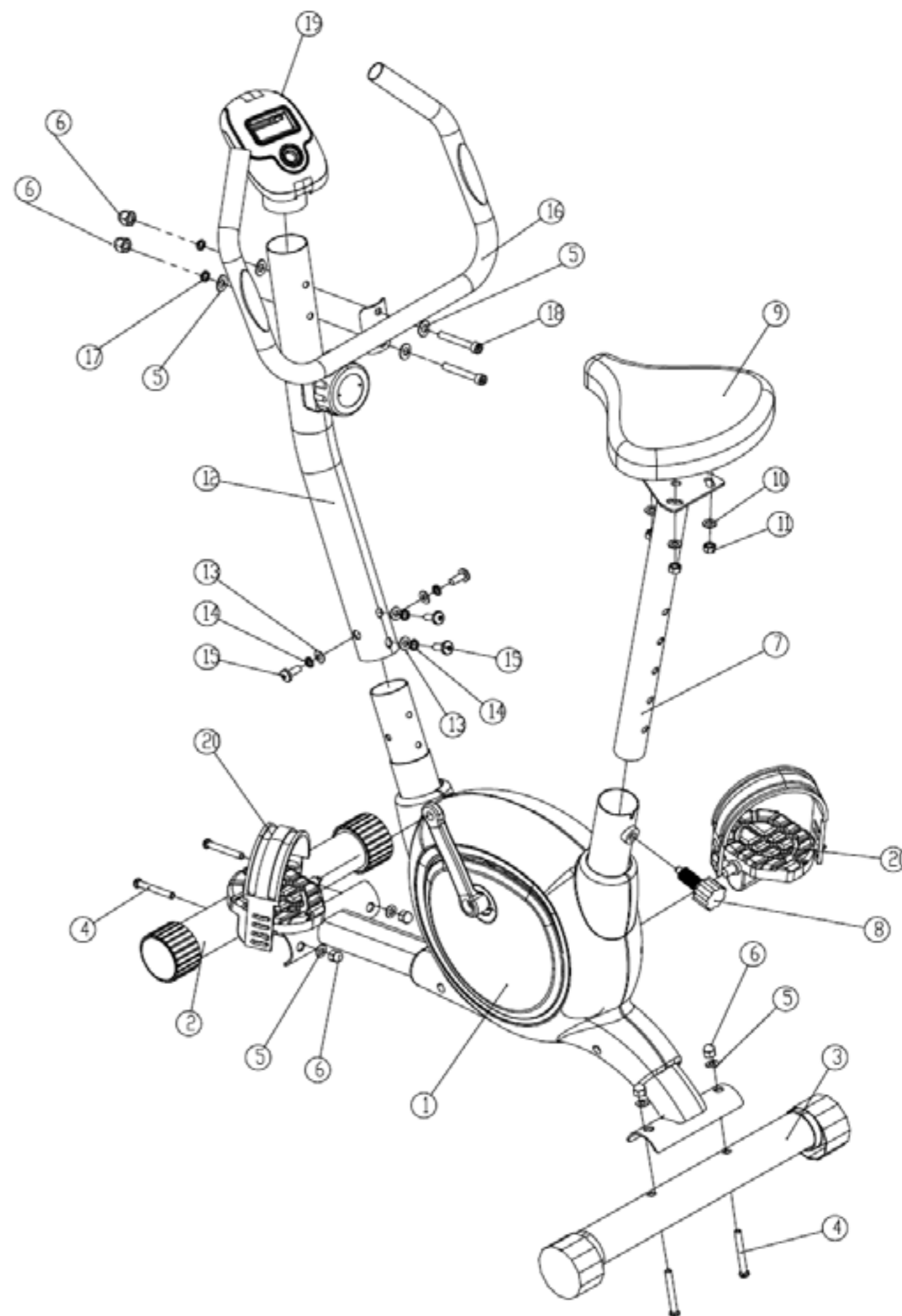
РИСУНОК-СХЕМА
